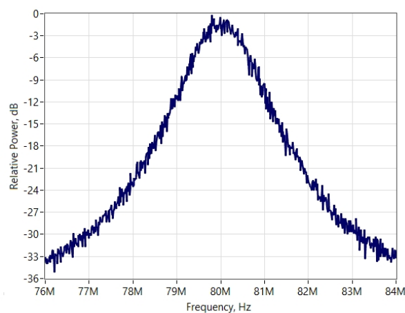
RF-line Spectrum
