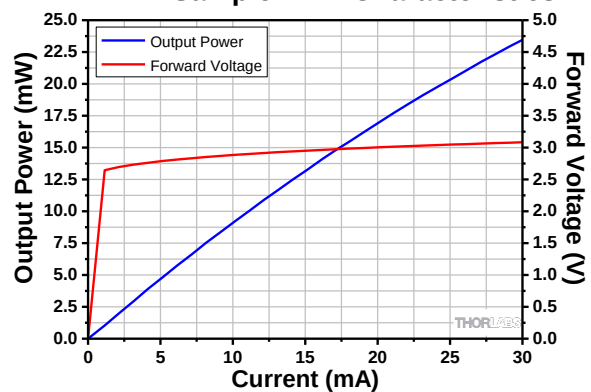
LEDW7E Sample L-I-V Characteristics
