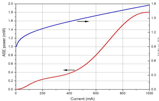
L-I-V curve
