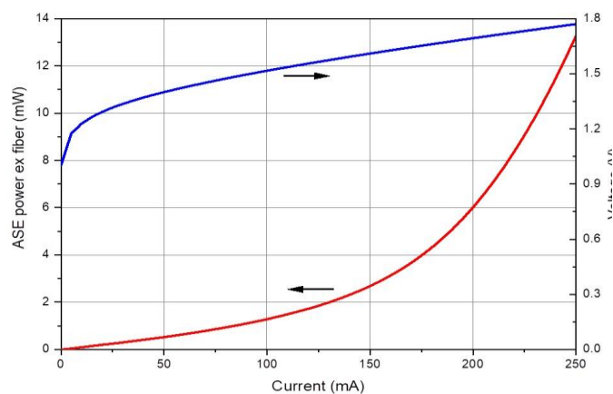
L-I-V curve
