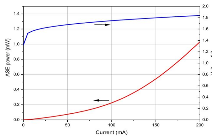
L-I-V curve
