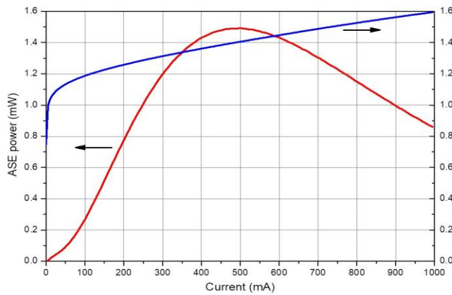
L-I-V curve
