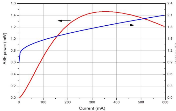
L-I-V curve
