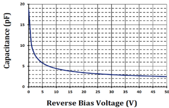
Capacitance vs. Reverse Bias Voltage Kapazität über Sperrspannung
