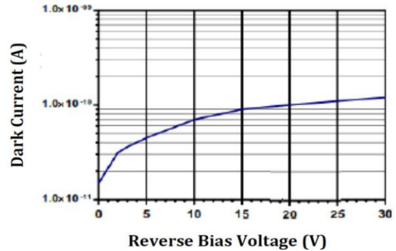
Dark Current vs. Reverse Bias Voltage Dunkelstrom über Sperrspannung
