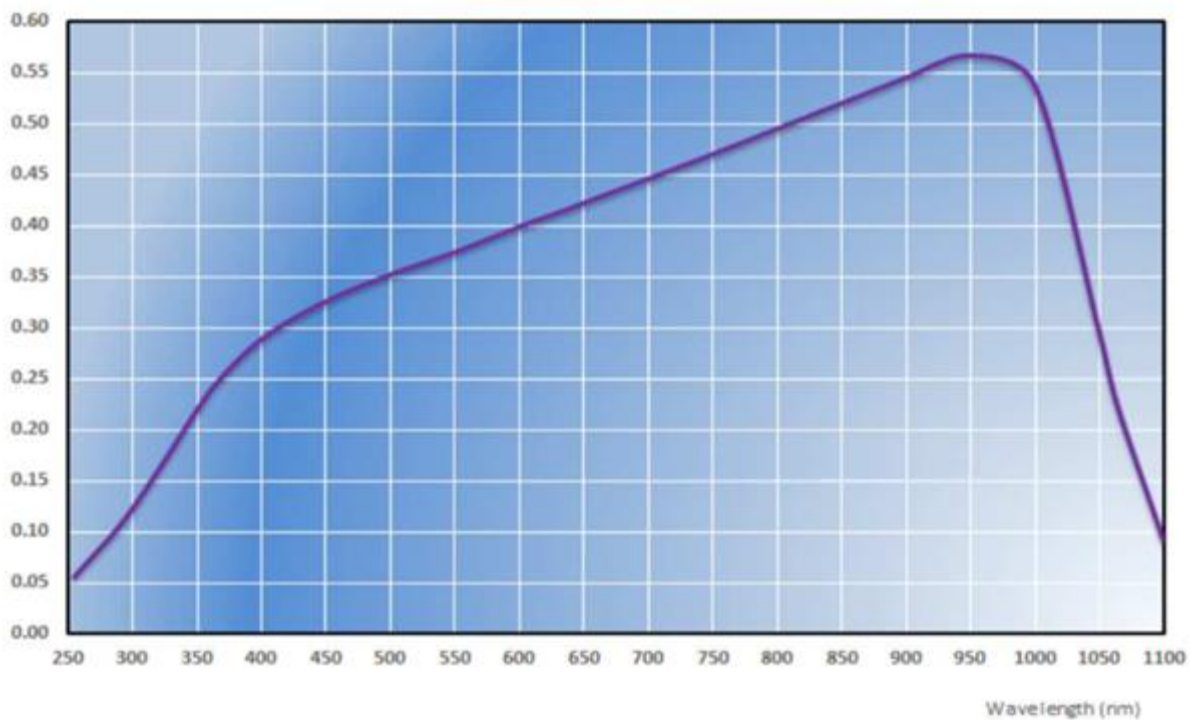
Typical Spectral Response Typische spektrale Empfindlichkeit
