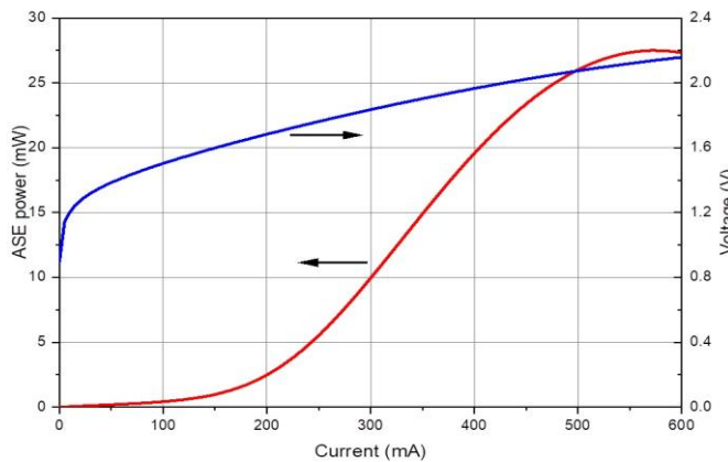
L-I-V curve
