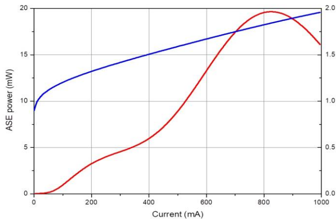
L-I-V curve
