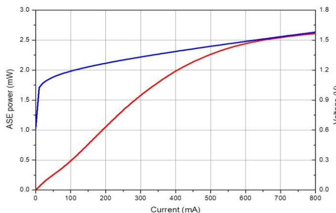
L-I-V curve
