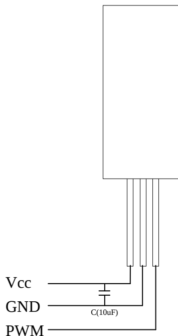
PWM mode
