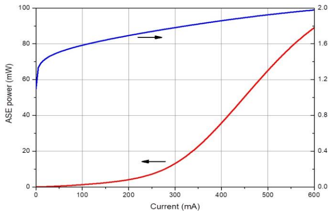
L-I-V curve
