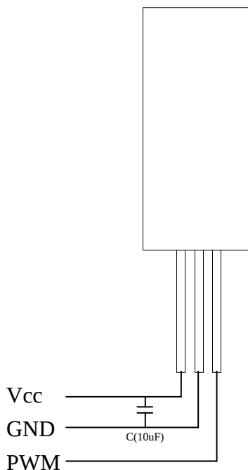
PWM mode
