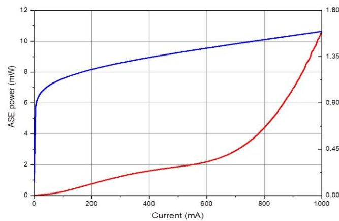
L-I-V curve
