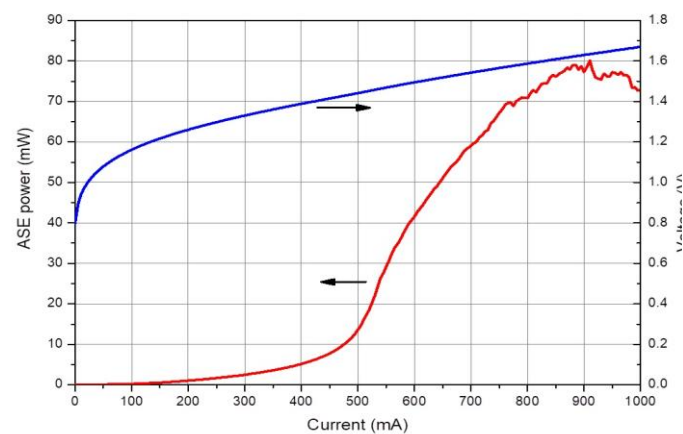
L-I-V curve
