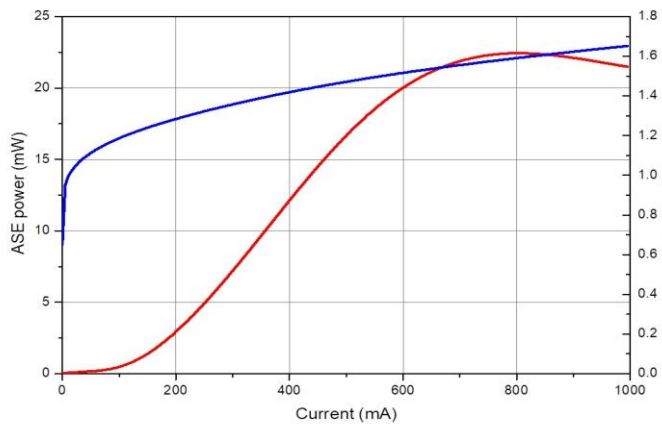
L-I-V curve
