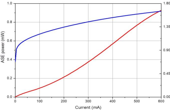
L-I-V curve
