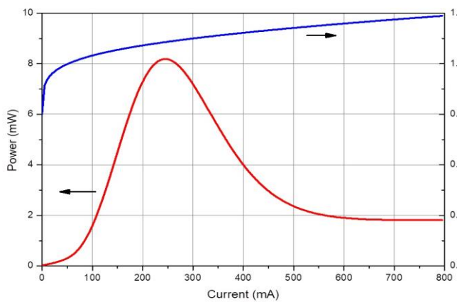
L-I-V curve
