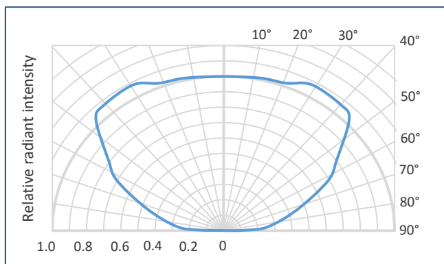
Lms1050LED-CS3020
