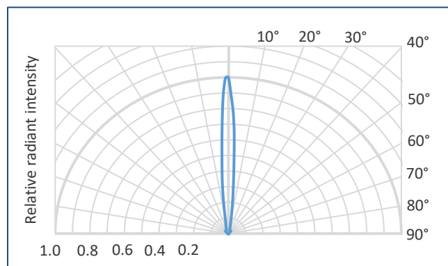
Lms1050LED-TEM-R
