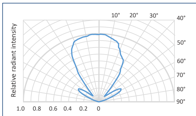
Lms1050LED-TEM
