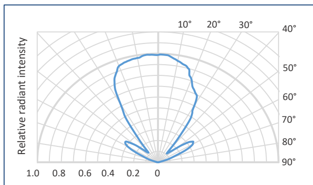
Lms20LED-TEM
