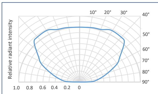
Lms20LED-CS3020
