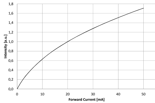
Intensity vs. Forward Current @ 25°C Strahlstärke über Flussstrom
