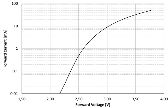
Forward Current vs. Forward Voltage @ 25°C Flussstrom über Flussspannung
