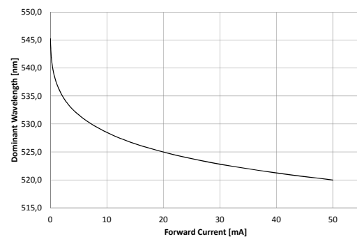
Dominant Wavelength vs. Forward Current @ 25°C Dominante Wellenlänge über Flussstrom
