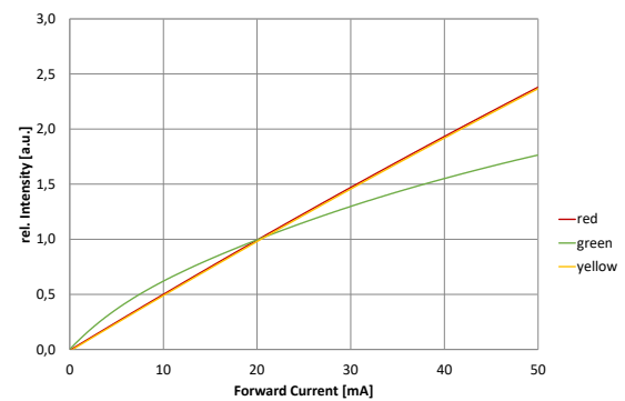
Luminous Intensity vs. Forward Current Rel. Lichtstärke über Flussstrom
