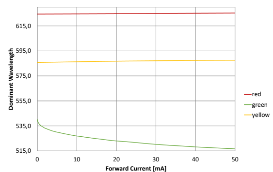
Dominant Wavelength vs. Forward Current Dom. Wellenlänge über Flussstrom
