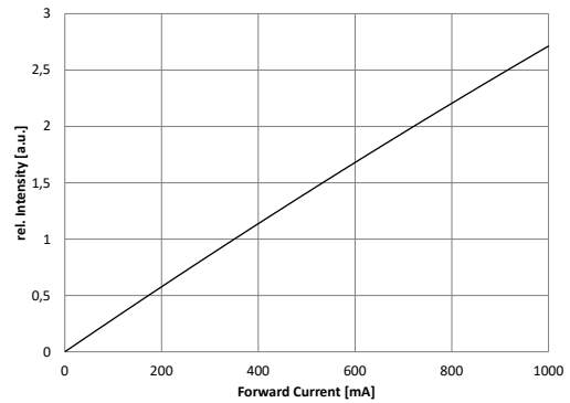
Intensity vs. Forward Current Strahlstärke über Flussstrom
