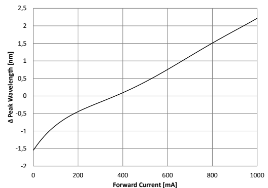
Shift Peak Wavelength vs. Forward Current Verschiebung der Wellenlänge über Flussstrom
