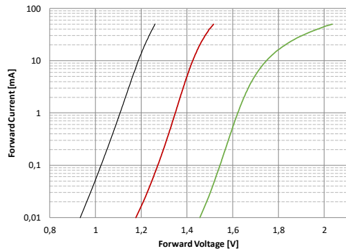
Forward Current vs. Forward Voltage Flussstrom über Flussspannung
