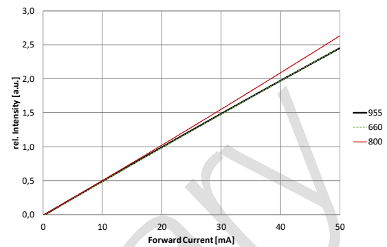
Radiant Intensity vs. Forward Current, Strahlstärke über Flussstrom
