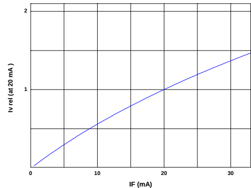
Intensity vs. Forward Current Lichtstärke über Flussstrom
