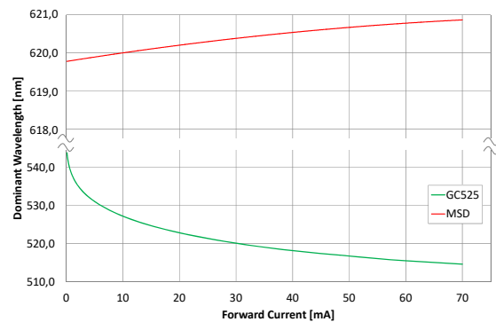
Shift Dominant Wavelength vs. Forward Current Verschiebung der Wellenlänge über Flusssstrom
