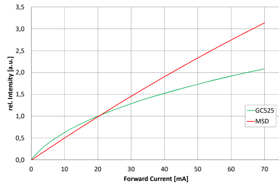
Intensity vs. Forward Current Lichtstärke über Flusssstrom
