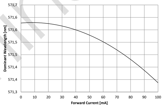
Forward Current vs. Shift dom. Wavelength Flussstrom gegen Verschiebung der Wellenlänge
