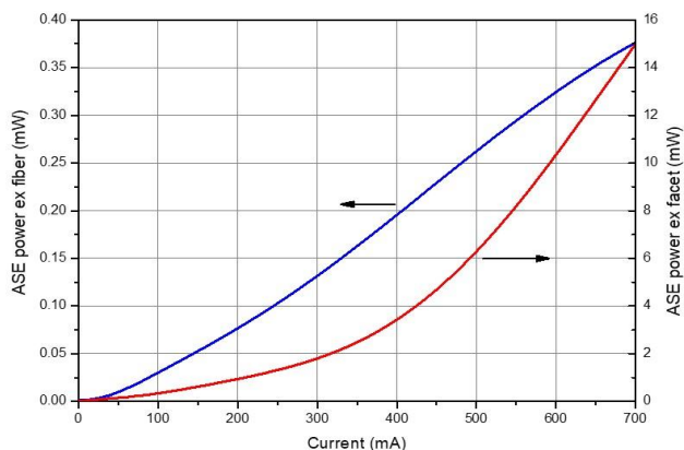
ASE power
