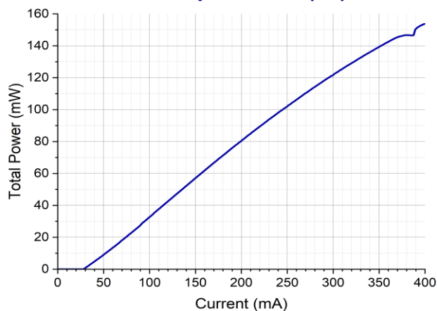
Total Output Power (L-I)
